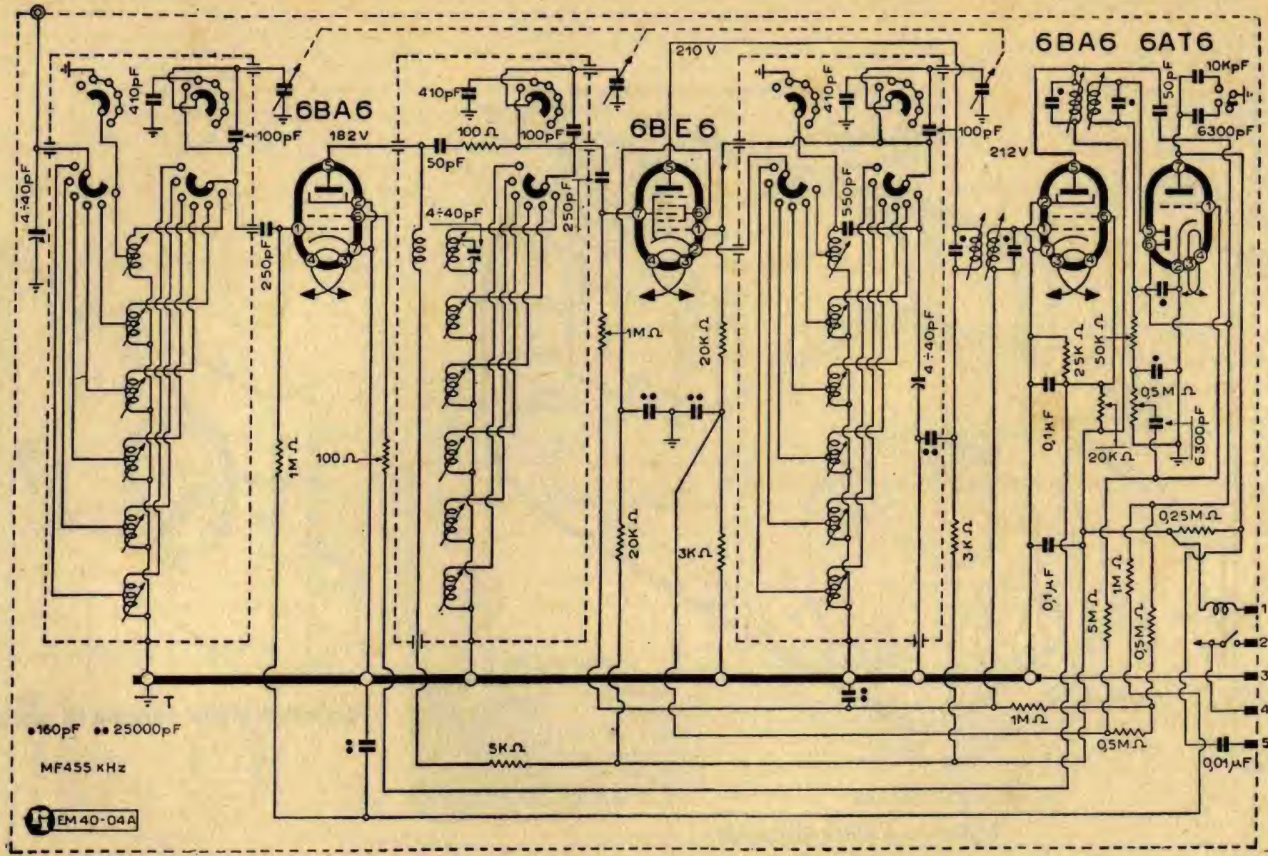
Lo schema elettrico dell'Autovox Mod. "RA 7/F., (sezione a)
